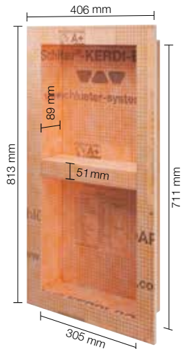
KB 12 N 305 711 A1 avec tablette intermédiaire
