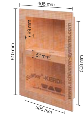
KB 12 N 305 508 A1 avec tablette intermédiaire
